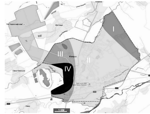
Рис. 1. Карта-схема кластерів засолення ґрунтів Калуша
