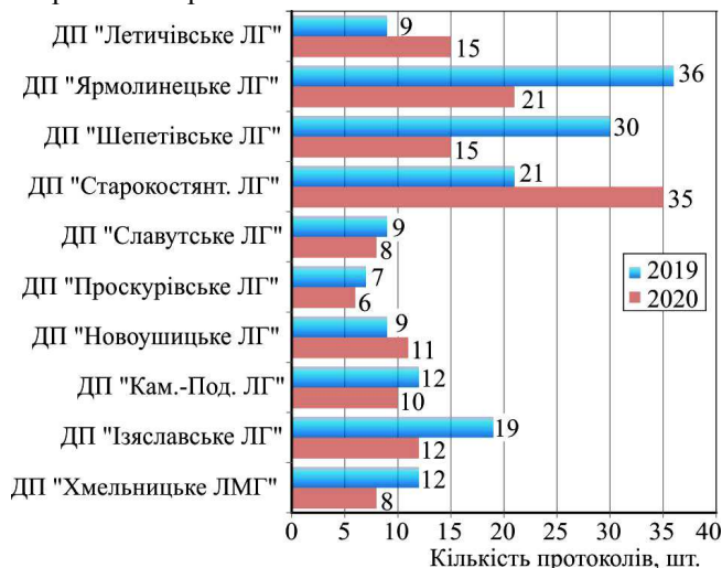
Рис. 4. Кількість складених протоколів для окремих лісових господарств Хмельницької області за 2019 і 2020 роки / Number of protocols drawn up for individual forestries of Khmelnytsky Region for 2019 and 2020
