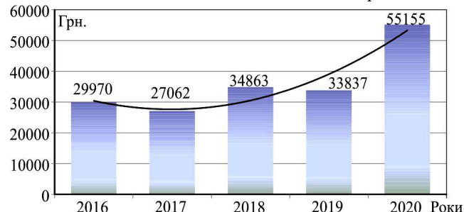
Рис. 3. Накладено штрафів на порушників правил полювання з 2016 по 2020 роки на території Хмельницької області, грн / Violators of hunting rules were fined from 2016 to 2020 in Khmelnytsky Region, hryvnia
