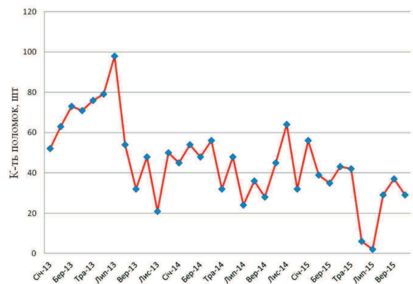
Рис. 5. Поломки двигуна
