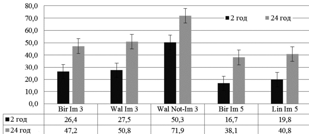
Рис. 3. Водопоглинання досліджених зразків, %
