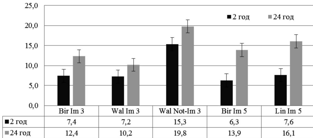
Рис. 4. Набрякання по товщині досліджених зразків, %
