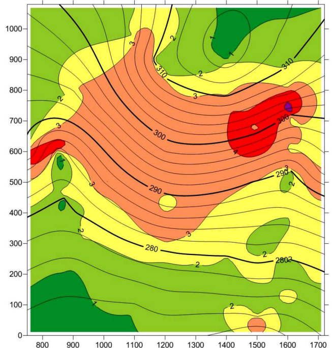
Рис. 2. Карта крутизни схилу (у градусах)
