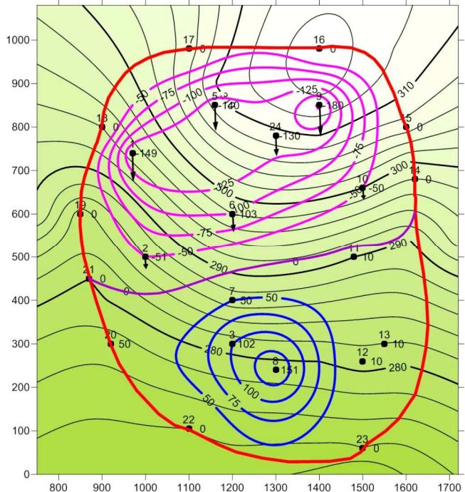
Рис. 3. Карта ізозміщень на зсувному схилі (у мм)
