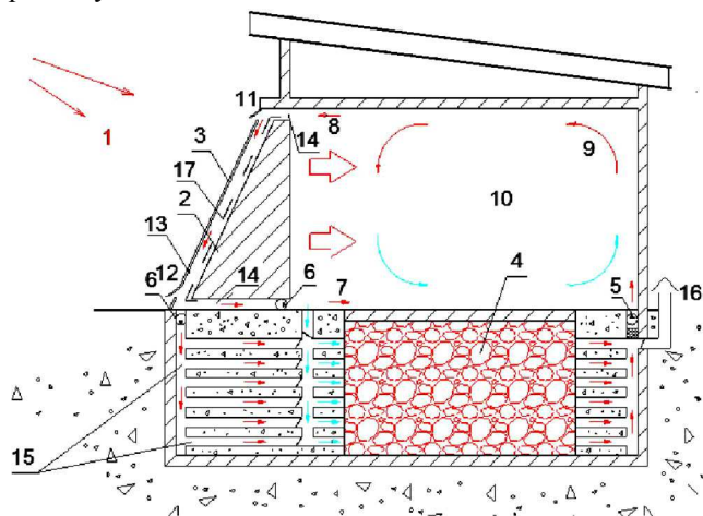
Рис. 1. Схема пассивної системи сонячного обігріву: 1) Сонце; 2) стіна Тромбе-Мішеля; 3) подвійне скління; 4) щебеневий акумулятор; 5, 6) вентилятори; 7) вхідний потік повітря; 8) висхідний потік повітря; 9) потік повітря, нагрітий в акумуляторі; 10) приміщення, що нагрівається; 11, 12) шибери у склінні; 13) проміжок між склінням; 14) циркуляційні канали у стінці Тромбе-Мішеля; 15) канали подавання повітря в тепловий акумулятор; 16) канал відведення повітря; 17) штора
