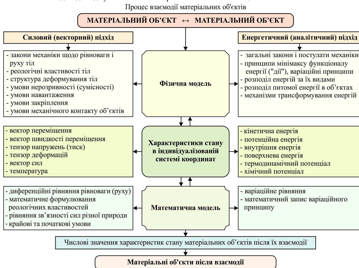
Рис. 1. Структурна схема силового та енергетичного підходів у моделюванні та визначенні стану матеріальних об'єктів
