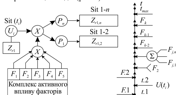
Рис. 3. Ситуаційна діаграма у вигляді ланцюга розгортання подій
