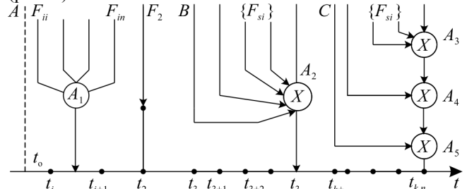
Рис. 5. Термінальна діаграма впливу факторів на режим об'єкта
