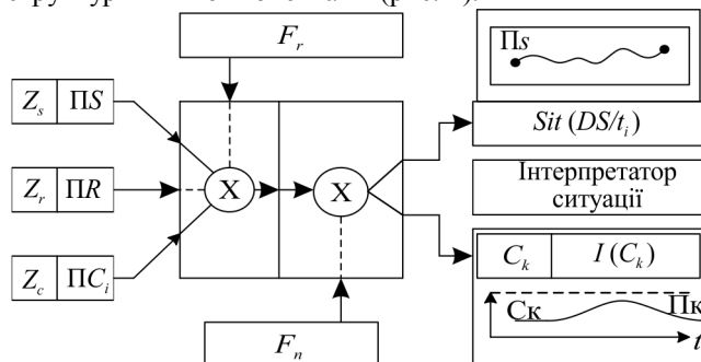
Рис. 1. Блок-схема структурних зв'язків
