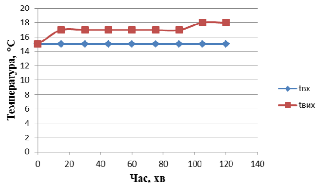
Рис. 3. Результати експериментальних досліджень геліопокрівлі без прозорого покриття для I_6 = 900 \text{ Вт} : t_{\text{вх}} – температура води на вході в геліопокрівлю, ^\circ\text{C} ; t_{\text{вих}} – температура води на виході з геліопокрівлі, ^\circ\text{C}
