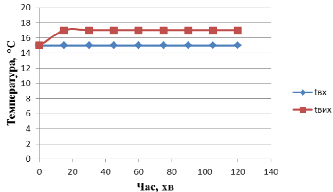
Рис. 2. Результати експериментальних досліджень геліопокрівлі без прозорого покриття для I_6 = 300 \text{ Вт} : t_{\text{вх}} – температура води на вході в геліопокрівлю, ^\circ\text{C} ; t_{\text{вих}} – температура води на виході з геліопокрівлі, ^\circ\text{C}
