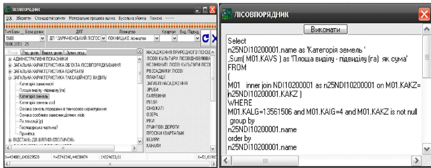
Рис. 4. Редактор "SQL" записи
