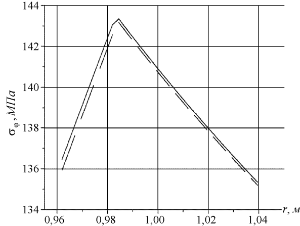
Рис. Розподіл колових пружно-пластичних напружень у порожнистій сфері
