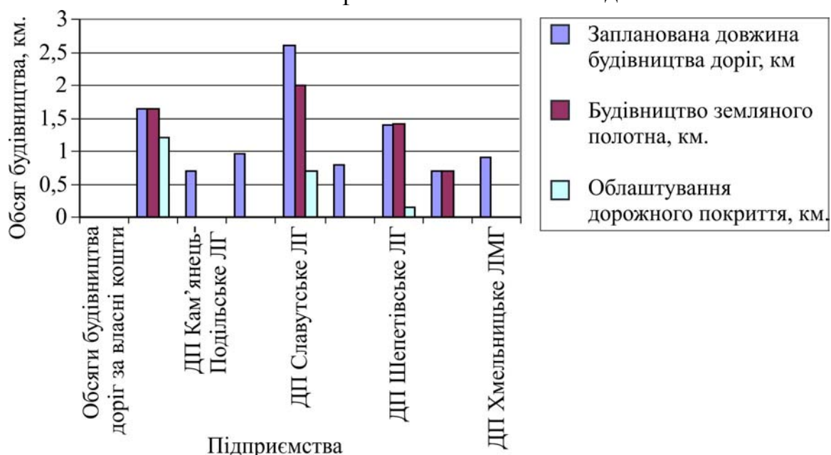
Рис. 1. Дані про фактичні та планові обсяги будівництва лісгосподарських доріг та доріг іншого значення за підприємствами лісопромислового виробництва Хмельницької обл.
