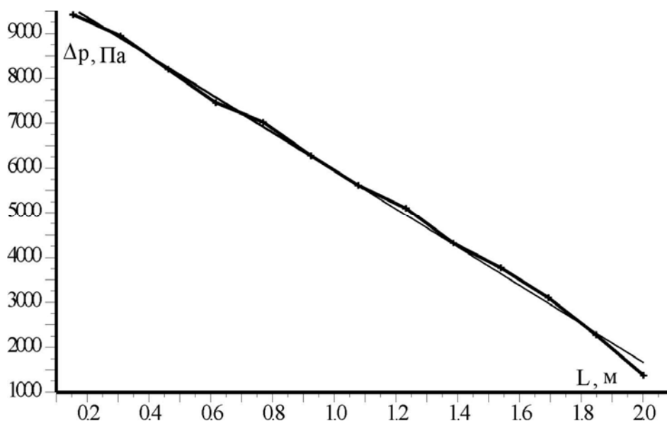
Рис. 3. Зміна гідравлічного опору шару по всій його довжині (висотою H = 70 \text{ мм} , довжиною L = 2 \text{ м} , кутом нахилу 2^\circ ): \Delta P – гідравлічний опір окремих ділянок шару, Па; L – довжина сушарки
