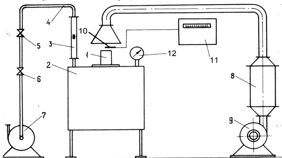
Рис. 1. Схема експериментальної установки: 1 – контейнер; 2 – ресивер; 3 – ротаметр; 4 – система трубопроводів; 5, 6 – регулювальний і запірний ventили; 7 – вакуумний насос; 8 – калорифер, 9 – вентилятор; 10 – термонара; 11 – потенціометр; 12 – вакууметр
