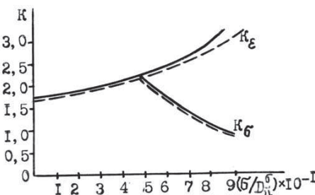
Рис. 3. Співставлення коефіцієнтів концентрації K для металевих зразків із отвором, отриманих за наведеною методикою аналітично (—) та експериментальним методом (---)
